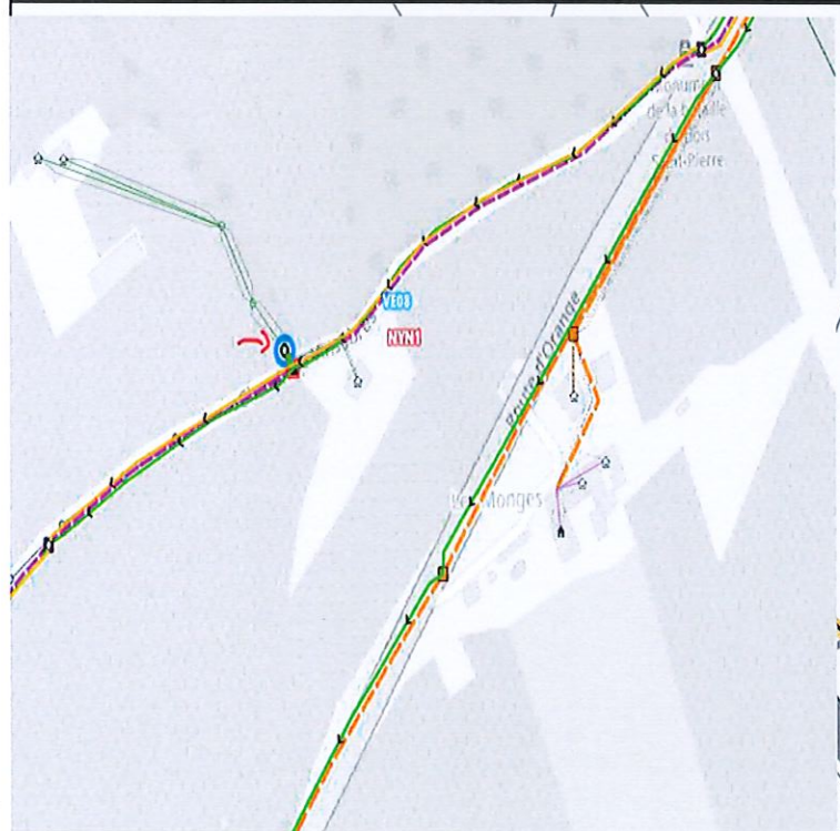
Carte d'implantation 1:1000
